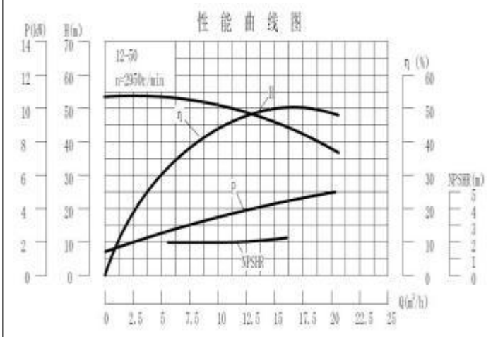
D12-50 泵技术数据 Technical Data
