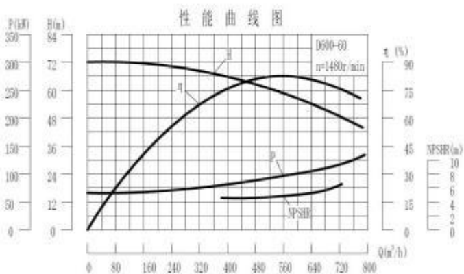
D600-60 泵技术数据 Technical Data
