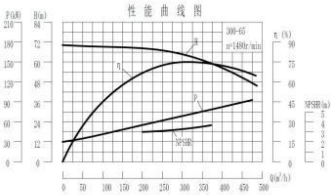
D300-65 泵技术数据 Technical Data
