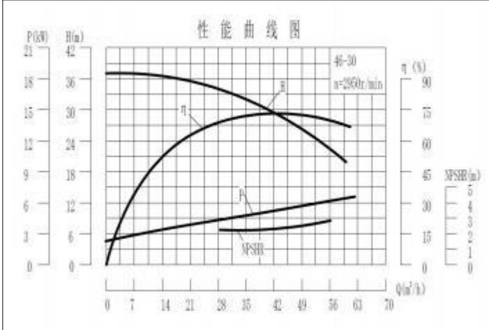
D46-30 泵技术数据 Technical Data
