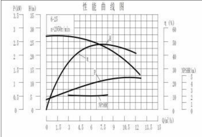
D6-25 泵技术数据 Technical Data
