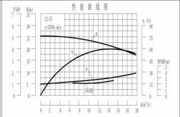
D12-25 泵技术数据 Technical Data
