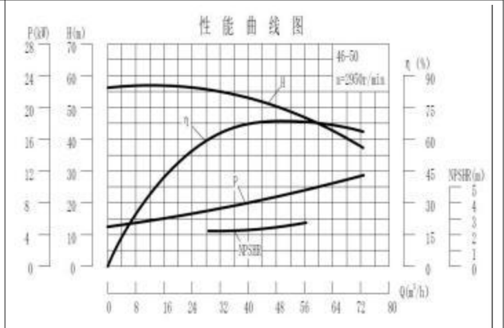
D46-50 泵技术数据 Technical Data
