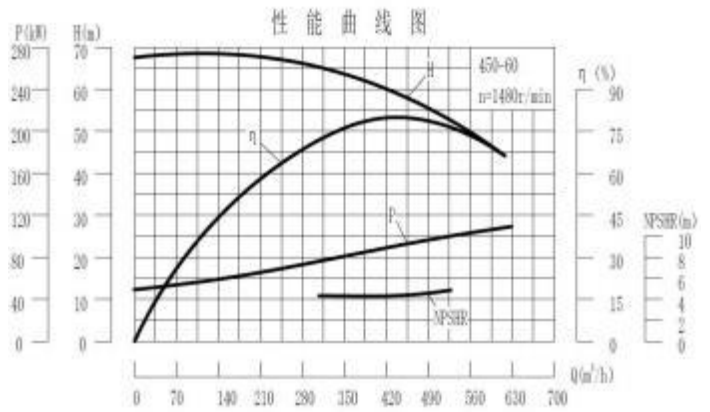
D460-60 泵技术数据 Technical Data
