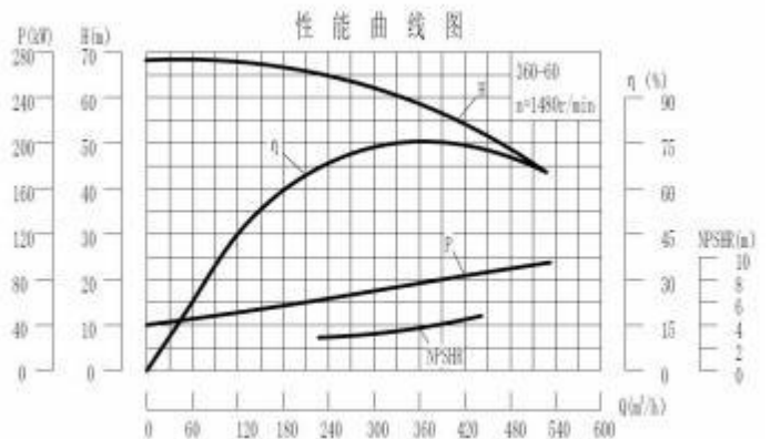
D360-60 泵技术数据 Technical Data
