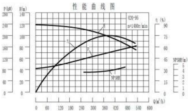
D420-95 泵技术数据 Technical Data
