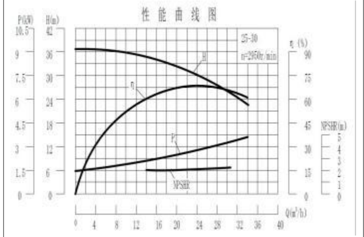
D25-30 泵技术数据 Technical Data
