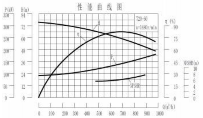
D720-60 泵技术数据 Technical Data
